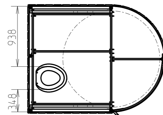
COUPE A-A
